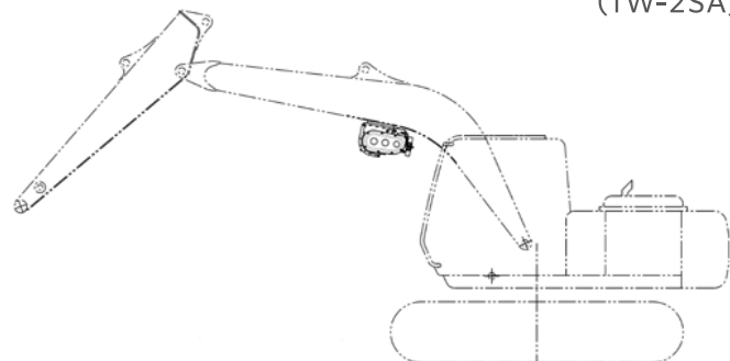
12t油圧ショベル架装状態 (TW-2SA)
